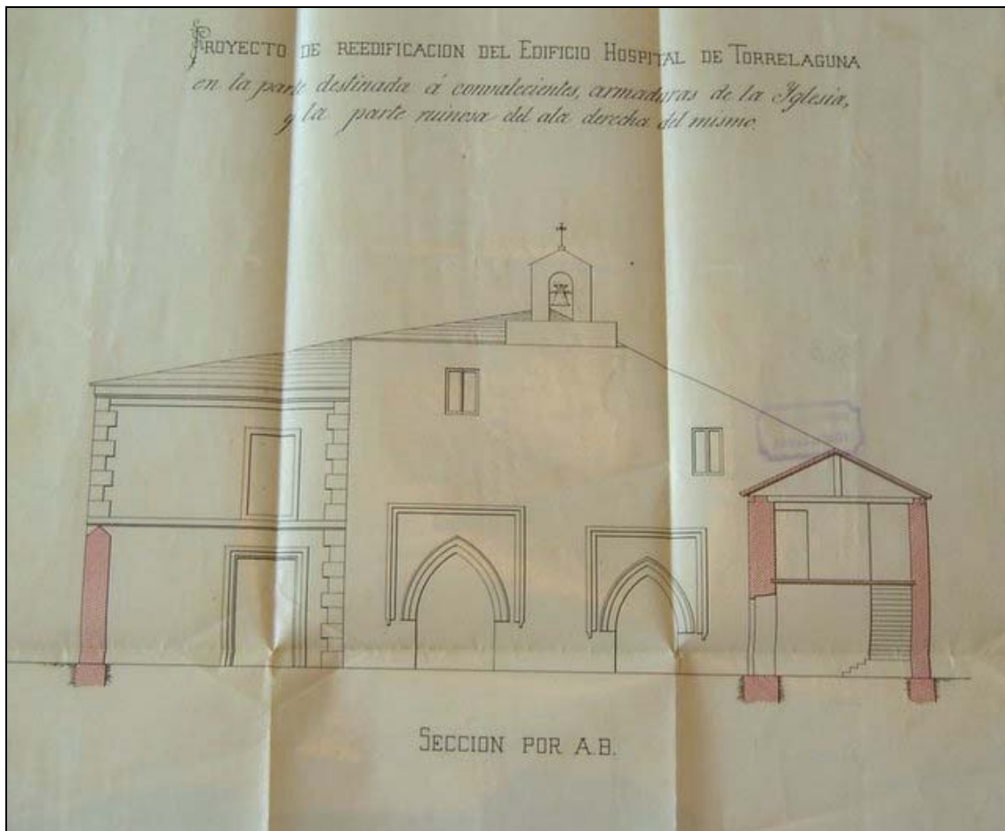
Proyecto a escala para la reparación del Hospital de la Santísima Trinidad, 1884, foto Mónica Vargas Guitart
