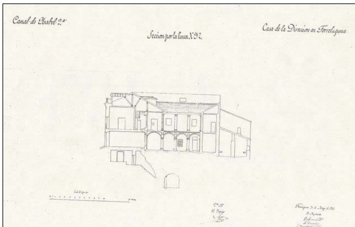
Sección de la Casa de la Dirección
