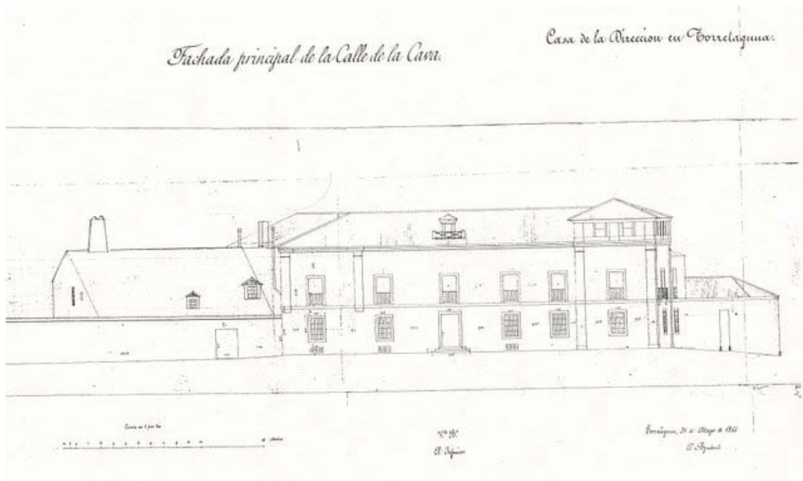
Plano de la fachada principal de la Casa de la Dirección, Francisco Echevarría
