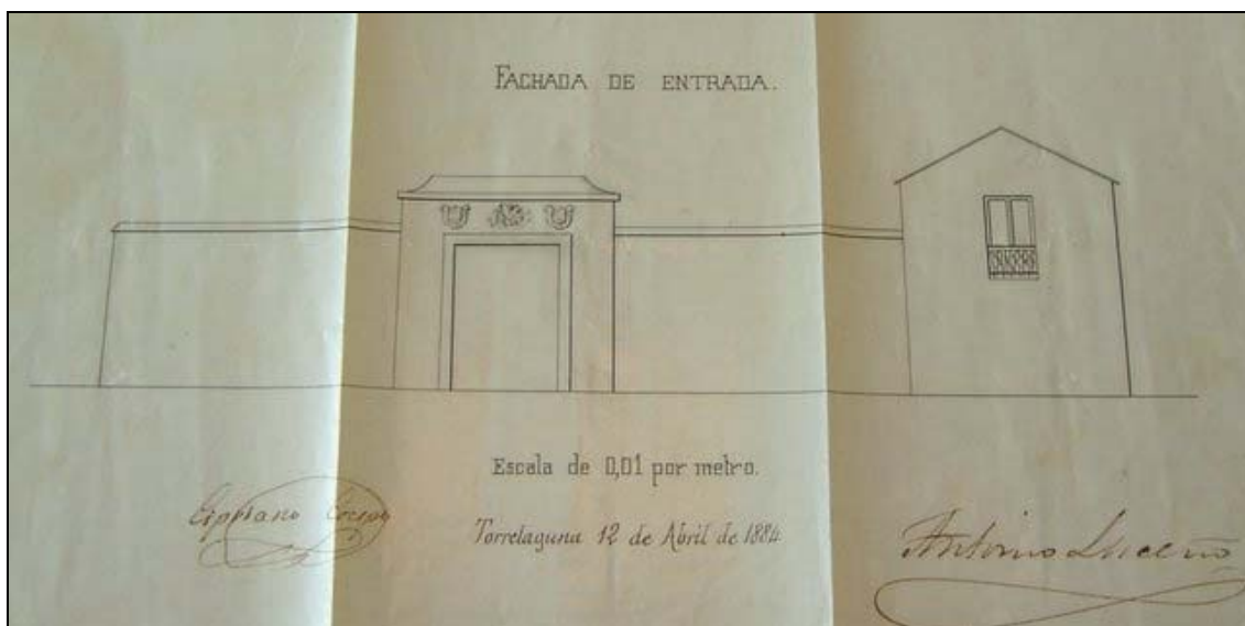
Plano de la Fachada de entrada del el Hospital de la Santísima Trinidad, 1884, foto Mónica Vargas Guitart
