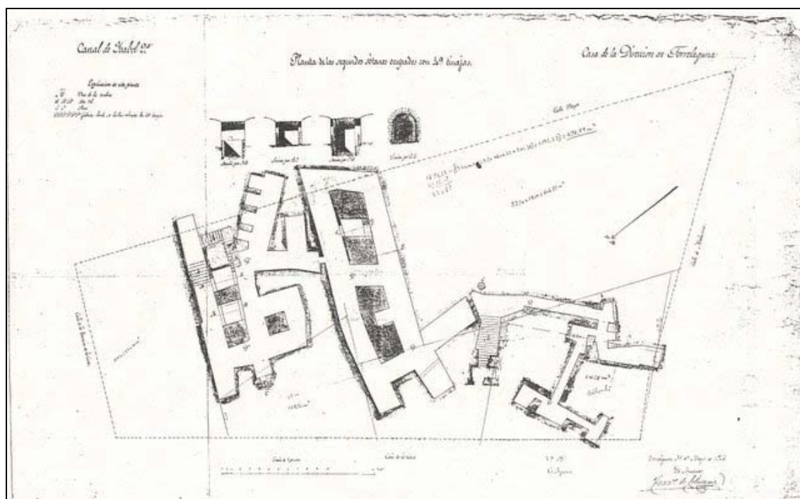
Plano de las cuevas de la Casa de la Dirección
