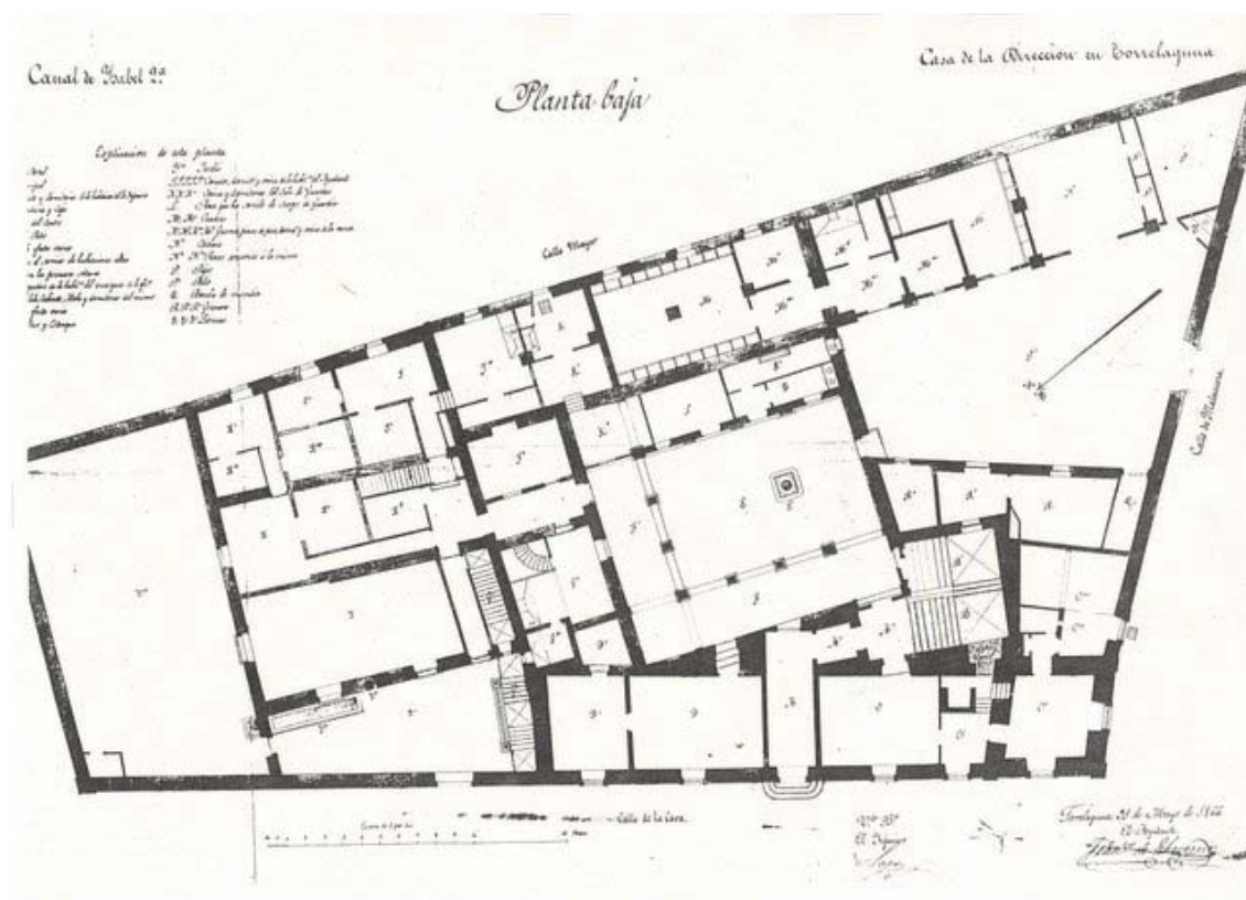
Plano de Francisco Echevarría de la Casa de la Dirección
