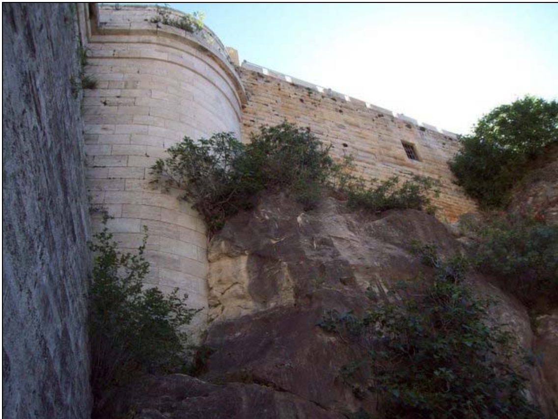
Detalle de la presa de El Pontón de la Oliva aguas abajo (Uceda, Guadalajara), foto: Sergio y Poli
